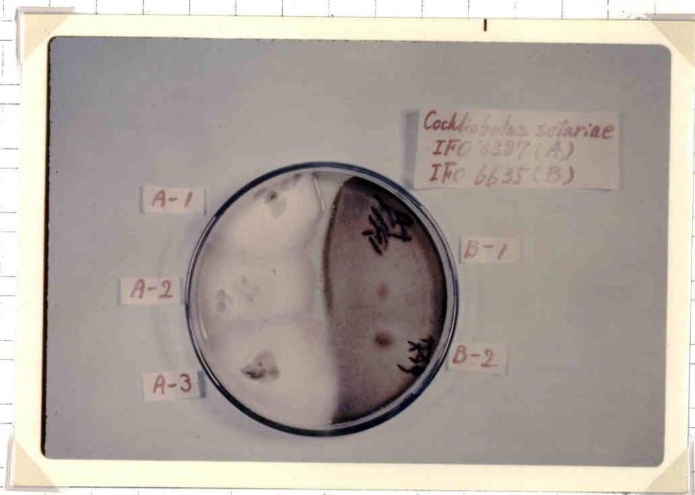
Cochliobolus setariae の IFO. 6387 菌と IFO. 6635 菌間の aversion 現象
