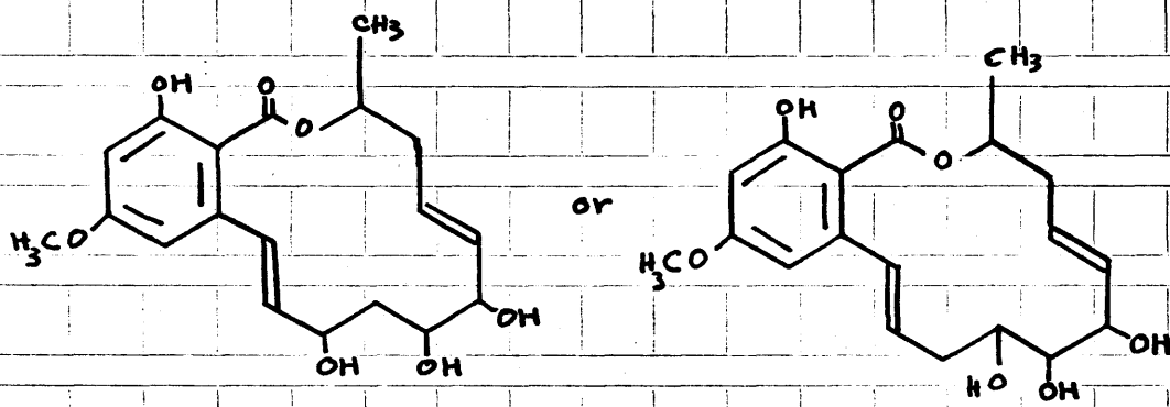
( P-C 19 化合物 )
