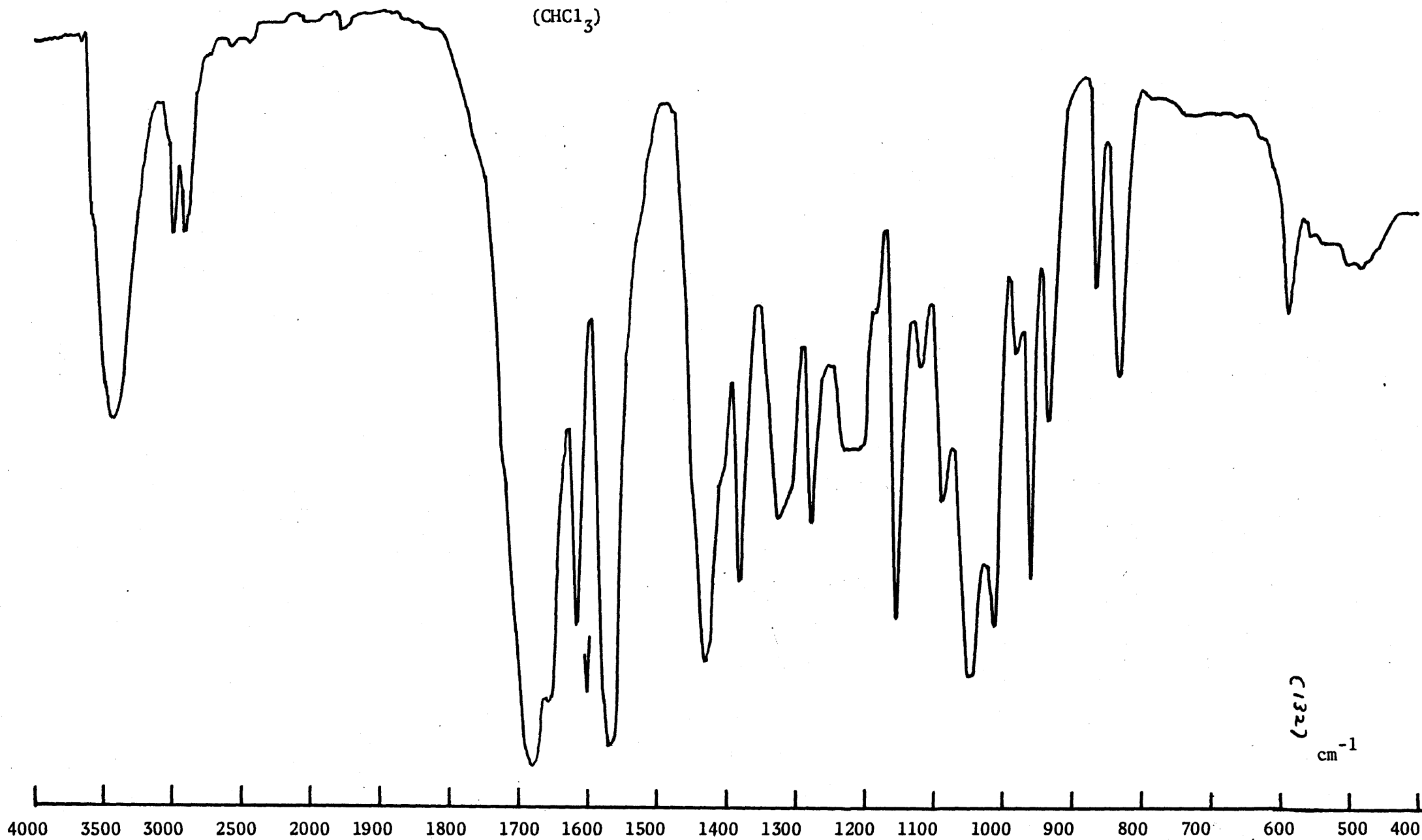
Fig. IR spectrum of radicinol.
