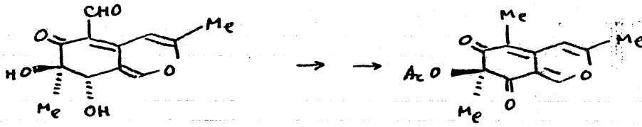
austdiol
