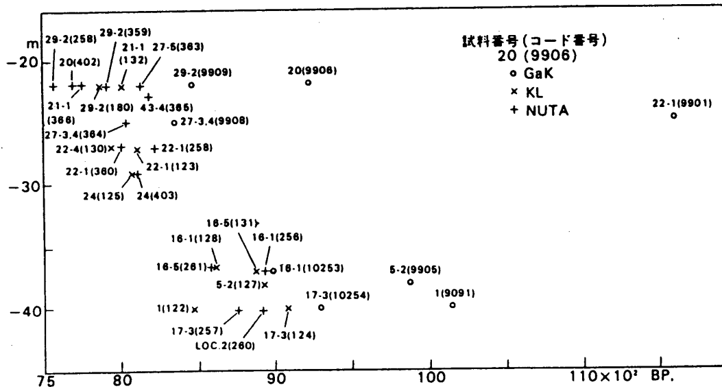
図1 ^{14}\text{C} 年代値と深度の分布図。 試料番号とコード番号が表1と対応する。
