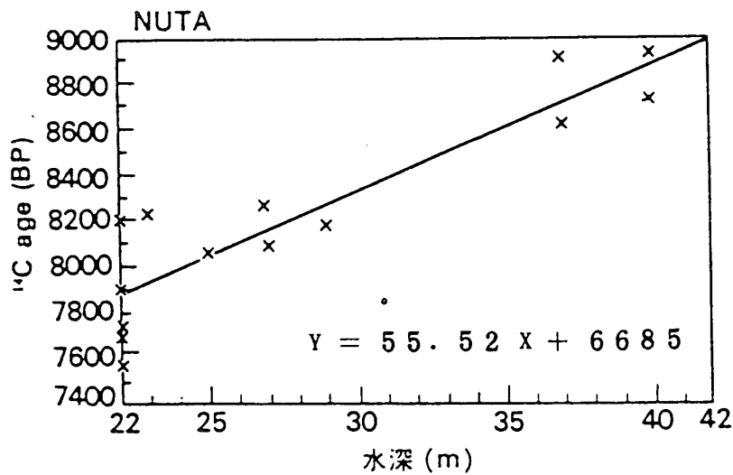
図2 名古屋大学加速器質量分析計による ^{14}\text{C} 年代値と水深との相関。
