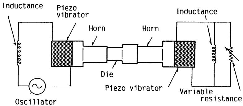
図4．機械的インピーダンス・電気的インピーダンス結合状況
