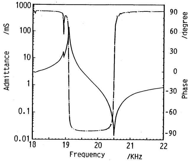
図 15. 周波数・アドミッタンス特性
