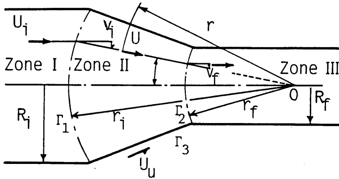
図 11. 表面進行波伝播の場合の可容速度場
