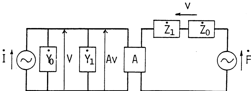
図14. 圧電振動子の等価回路
