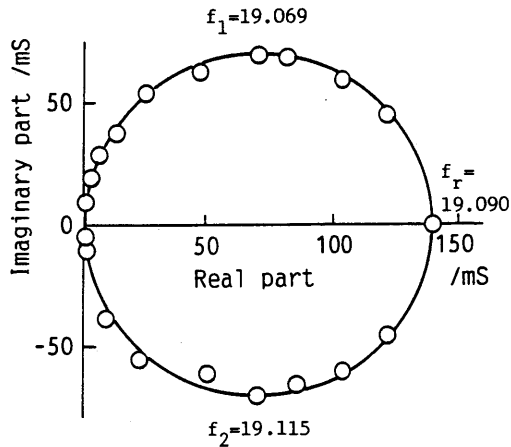
図 16. アドミッタンスループ
