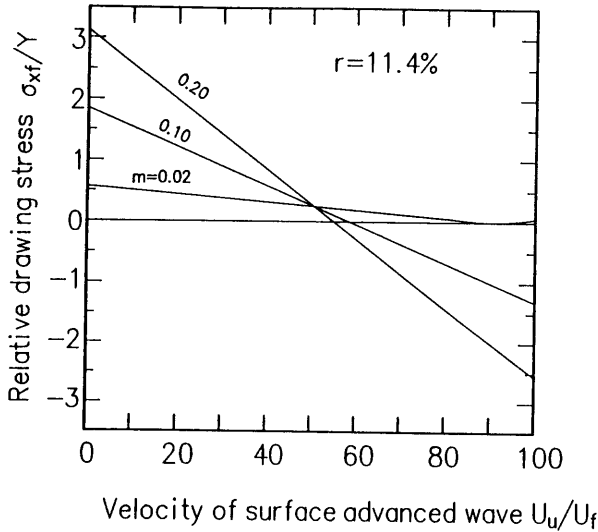
図12. 引抜き応力・進行波 伝播速度線図 (摩擦応力を変えた場合)
