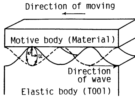
図3．表面進行波の伝播
