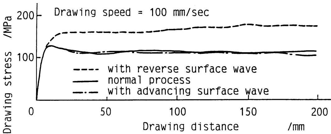
図10．引抜き応力・行程線図（引抜き速度 = 100 mm/sec）
