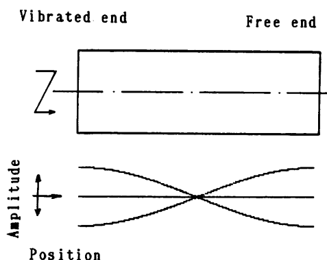
図1. 定在波
