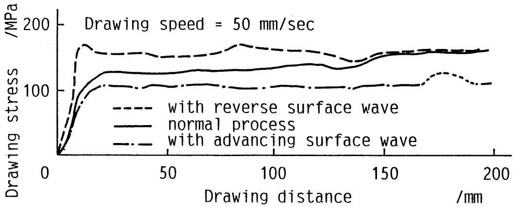
図9．引抜き応力・行程線図（引抜き速度 = 50 mm/sec）
