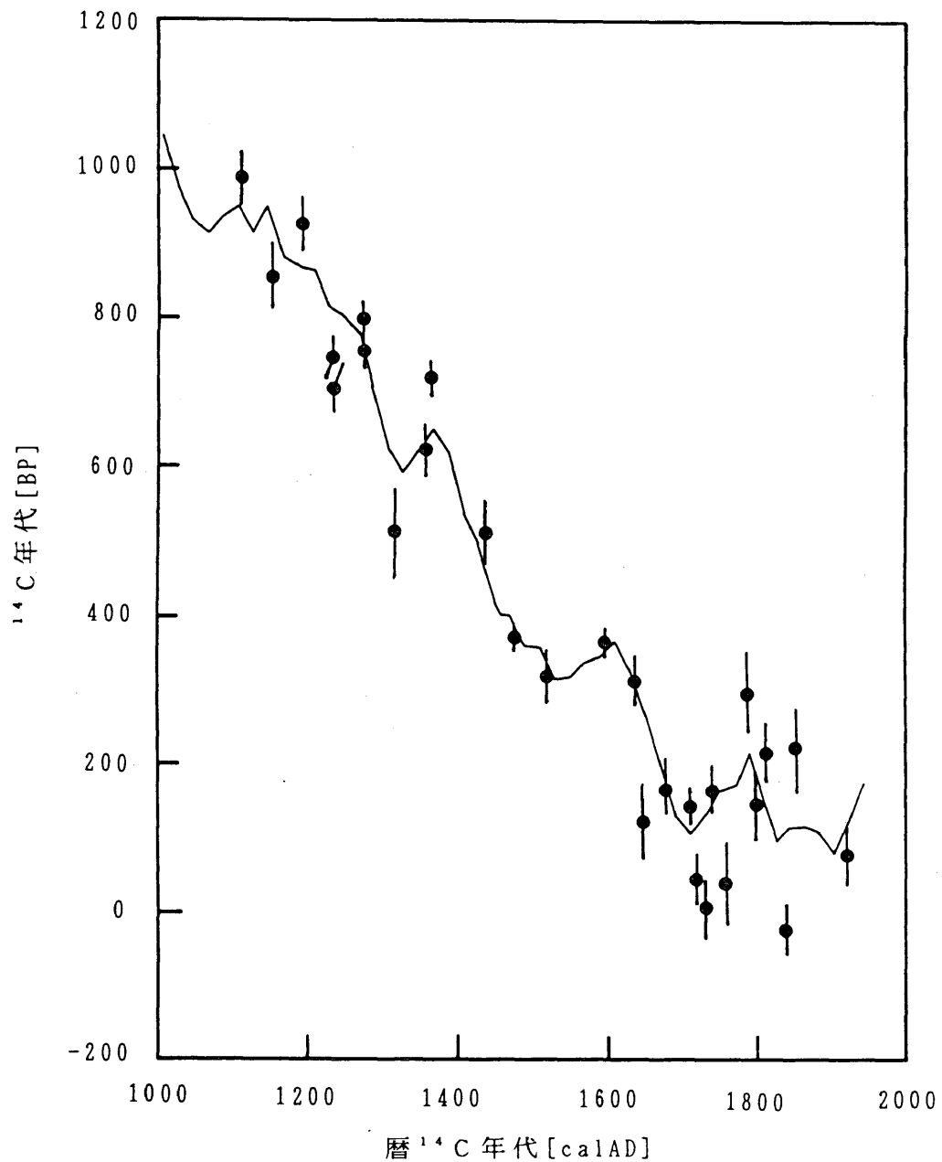
図1. 木曾ヒノキ年輪試料の暦年代と ^{14}\text{C} 年代
