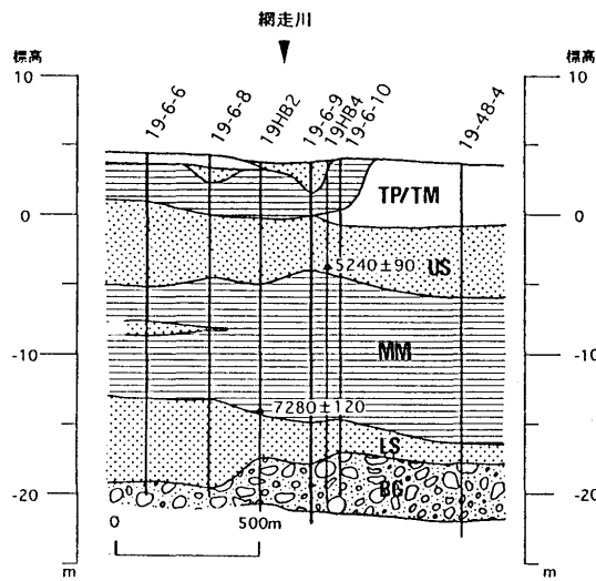
図4 19線沿いの地質断面図
