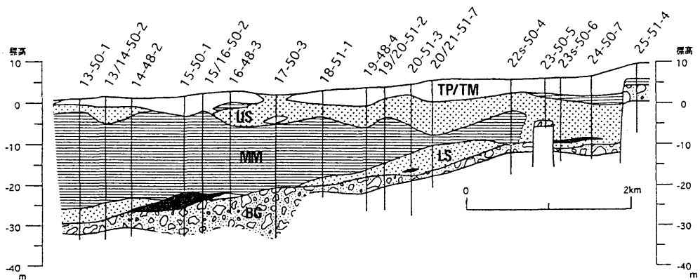
図5 低地縦断方向の地質断面図
