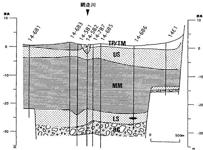
図3 14線沿いの地質断面図
