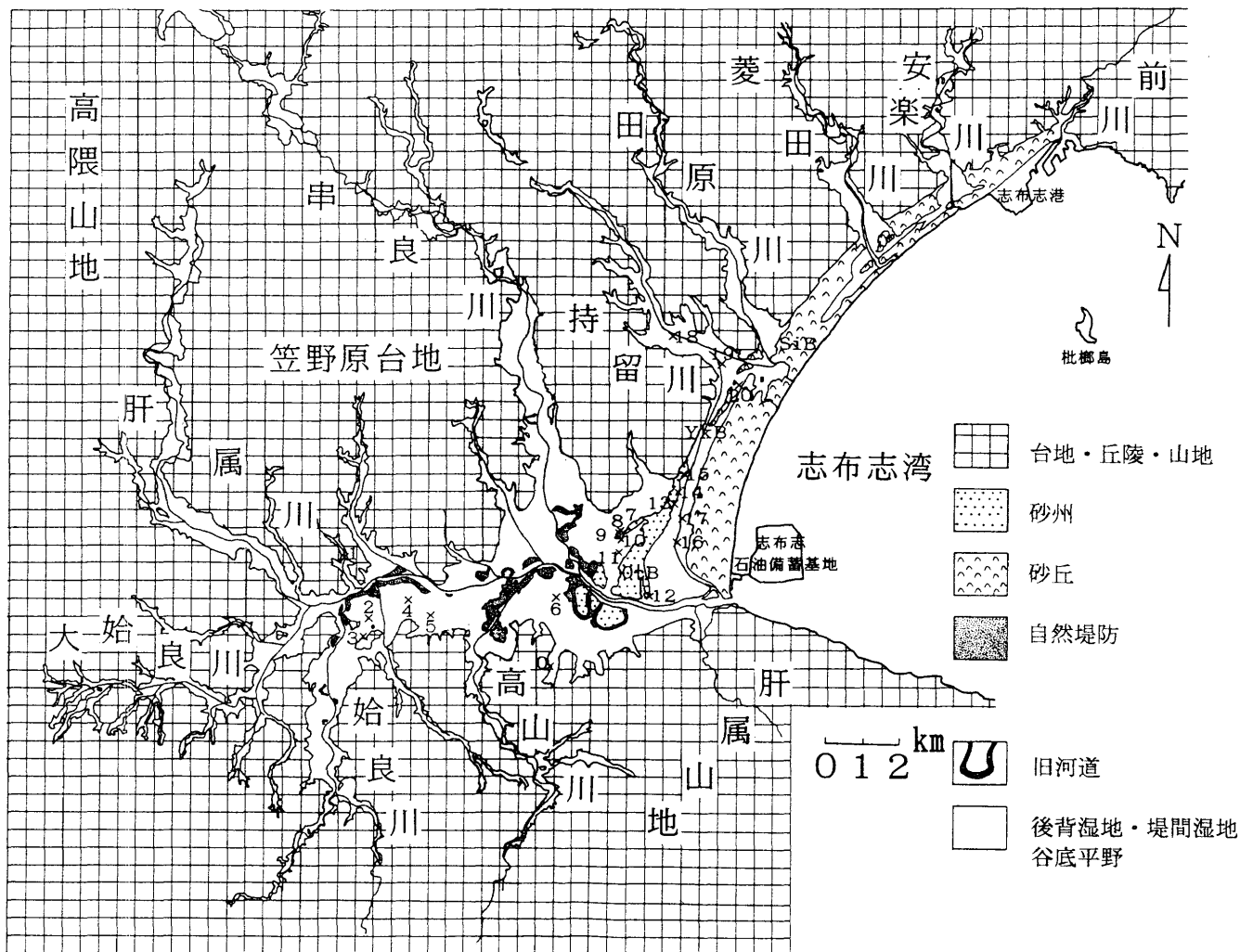
第2図 肝属平野の地形分類図
