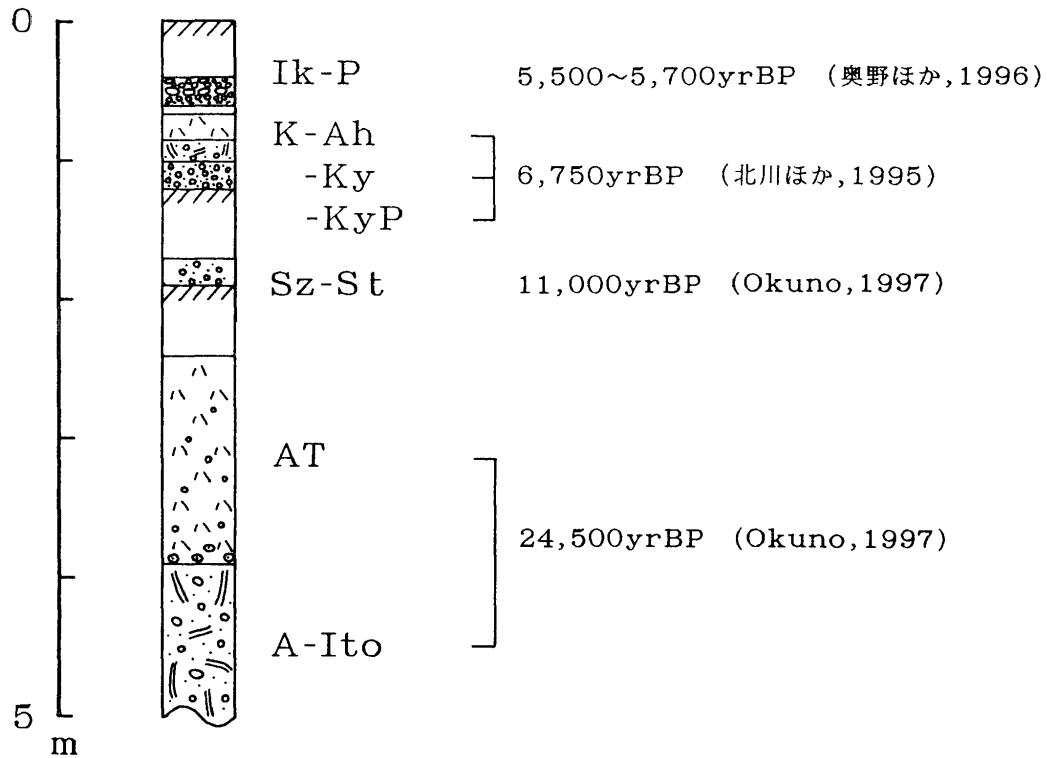
第3図 Loc.0におけるテフラ柱状図
