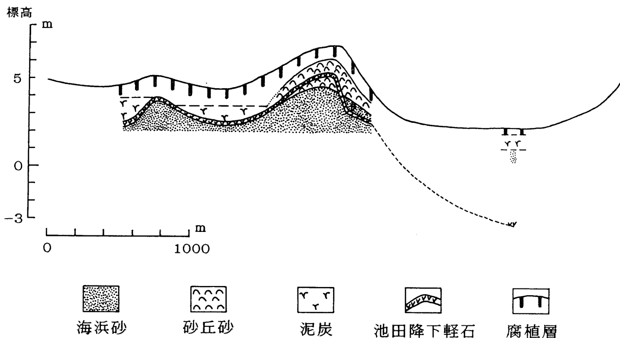
第 5 図 大塚砂州断面図
