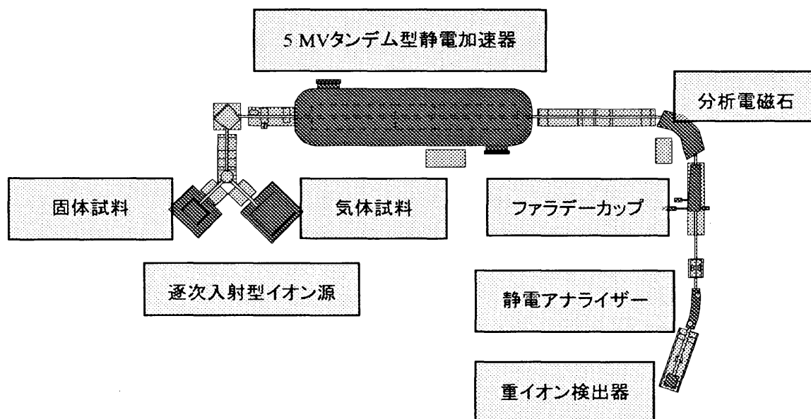
図 1 ペレトロン加速器質量分析計
