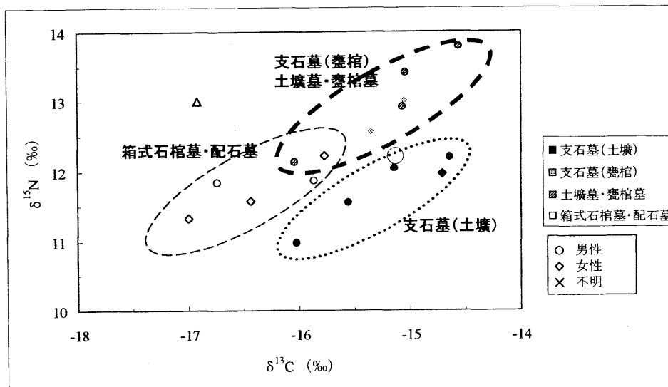
図4 時期別・男女別の \delta^{13}\text{C} ・ \delta^{15}\text{N}
