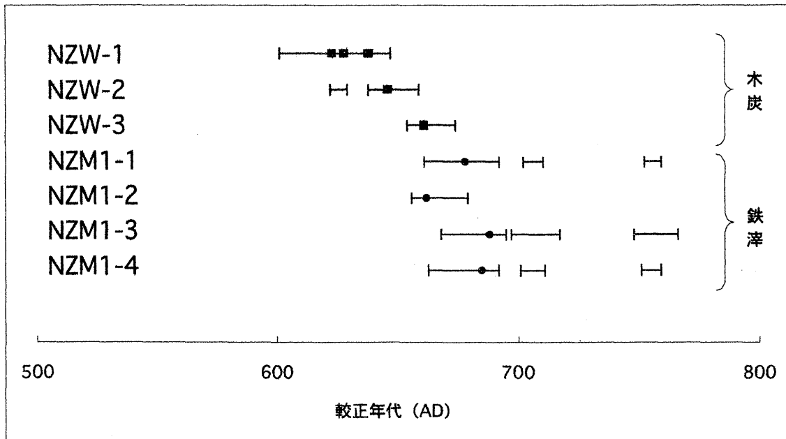
図2. 木炭および鉄滓試料の 14 C年代測定の結果の比較
