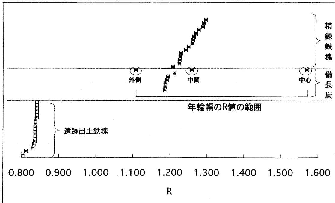
図 1. 精錬実験に用いた試料の ^{14}\text{C} 年代測定の結果の比
