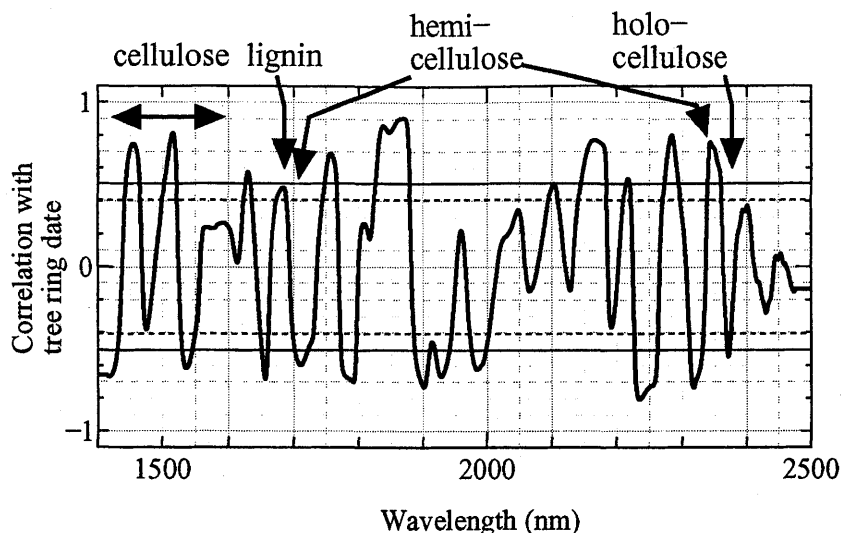
図 5: 波長 1400–2500nm での二次微分スペクトルと年輪年代の単相関。水平線は有意水準 0.1%(実線) および 1%(点線)。 Figure 5: Correlation function between tree-ring dates and second derivative spectra. Horizontal lines show significance level at 0.1% (solid) and 1% (dotted).
