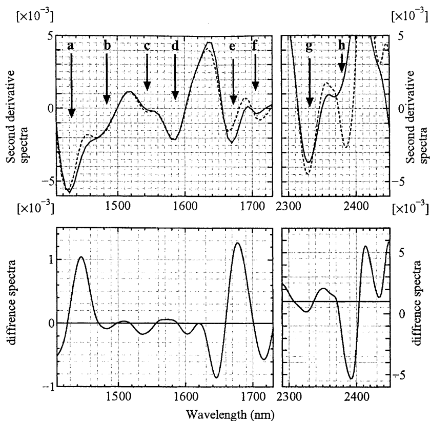
図 4: 古建築材 (AD7 世紀) の二次微分スペクトル (上). 実線は古文書資料. 和紙の年代は天保 2 年 (1645) および元和元年 (1615). 点線は現代の年輪試料 (AD1950). 下図は差スペクトル (1 式参照).
