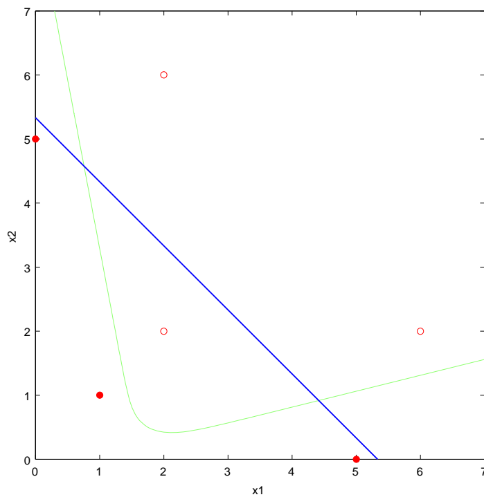
図 2: 第 6 回 演習問題 問 2 決定境界の比較 (Widrow-Hoff とニューラルネットワーク)
