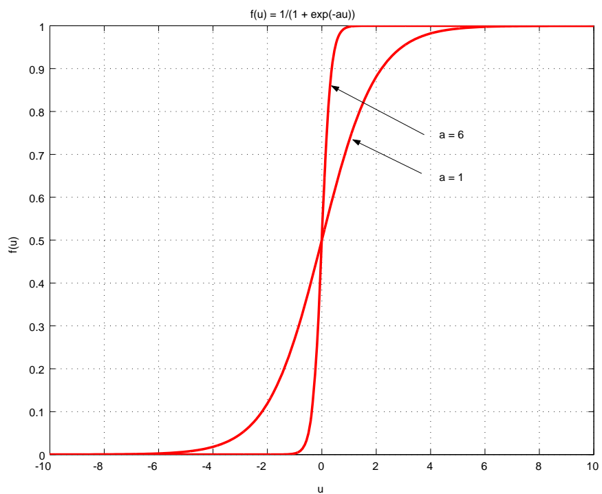
図 1: Sigmoid 関数 (Logistic 関数)
