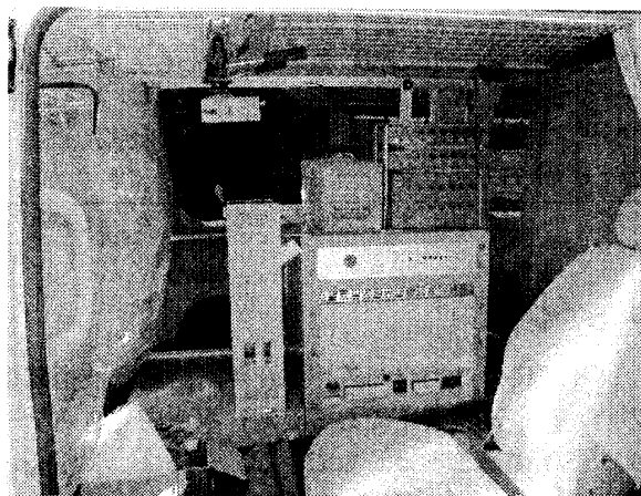
図 8: 後席（無停電電源装置とマイクアンプ
