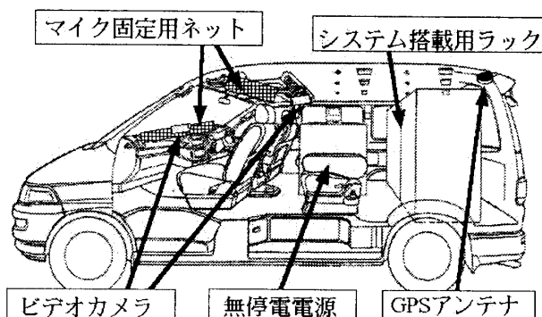
図 4: 収集用車両の概要
