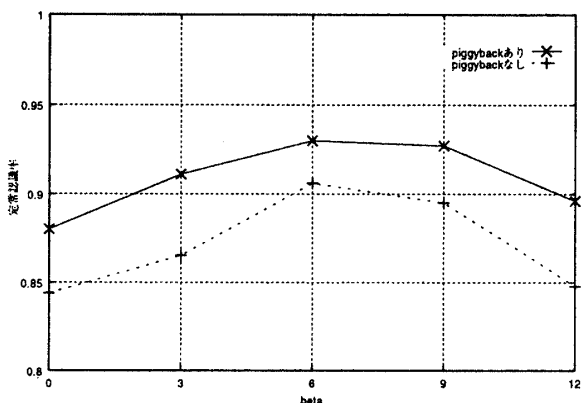
図 10: 各 \beta 値における定常認識率 ( lbr = 20, msr = 20 )
