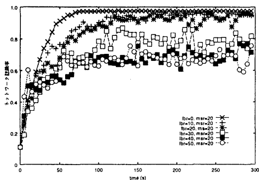
図 4: msr=20 に対するネットワーク認識率の推移
