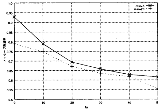
図 8: 各条件下のメッセージ到達率
