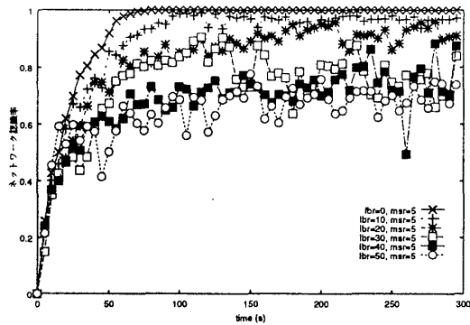
図 3: msr=5 に対するネットワーク認識率の推移
