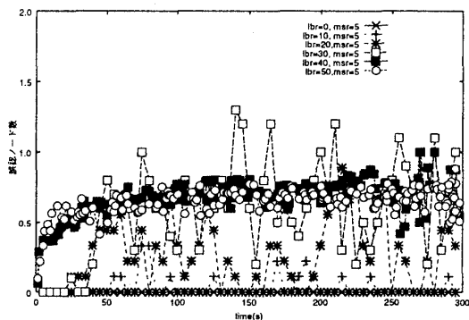
図 5: msr=5 に対する誤認ノード数の推移
