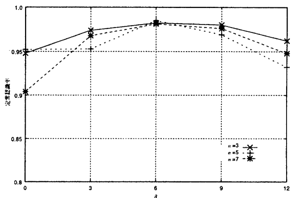
図 12: lbr=10, msr=20 のときの定常認識率
