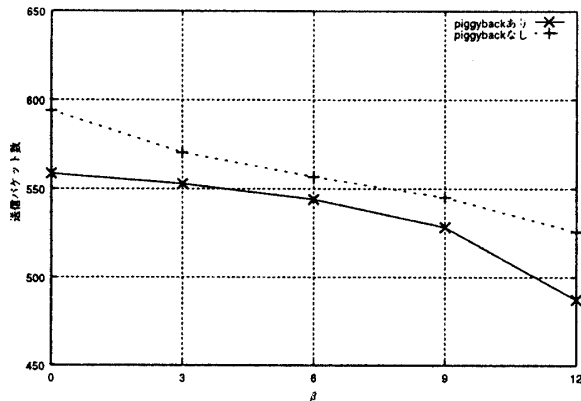
図 9: 各 \beta 値における総送信パケット数 ( lbr = 20, msr = 20 )
