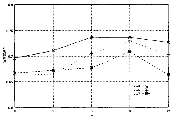
図 14: lbr=40, msr=20 のときの定常認識率
