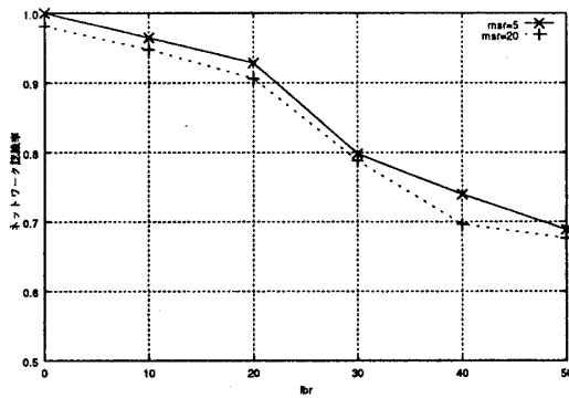
図 7: 各条件下の定常認識率
