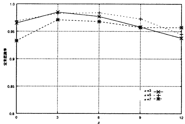
図 11: lbr=10, msr=5 のときの定常認識率
