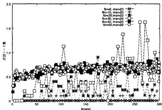
図 6: msr=20 に対する誤認ノード数の推移
