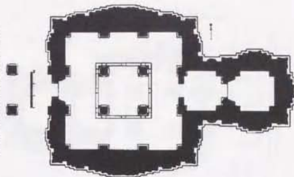
Fig. 205. Hedatale Nagaresvara temple plan.
