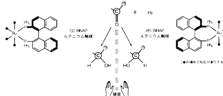
BINAP-ルテニウム触媒を用いた水素化反応の例(模式図)
