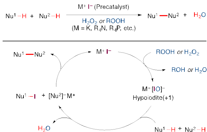
図1: 無機ヨウ素化合物/過酸化物を用いる触媒的酸化システム
