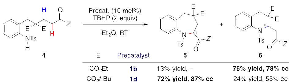
図6: \alpha -酸化 versus \beta -酸化
