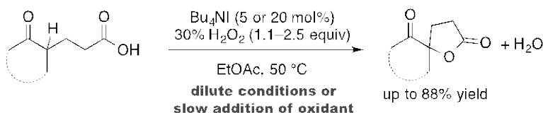
図4: 次亜ヨウ素酸塩を触媒として用いる脂肪族オキソカルボン酸のオキシラクトン化反応
