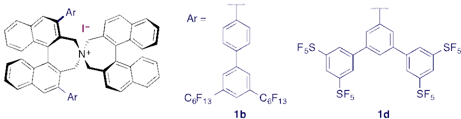
図7: 位置及びエナンチオ選択的酸化的アミノ環化反応を鍵とする6,7員環合成
