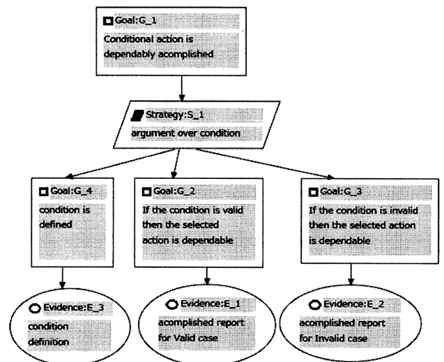
図2 条件分解戦略
