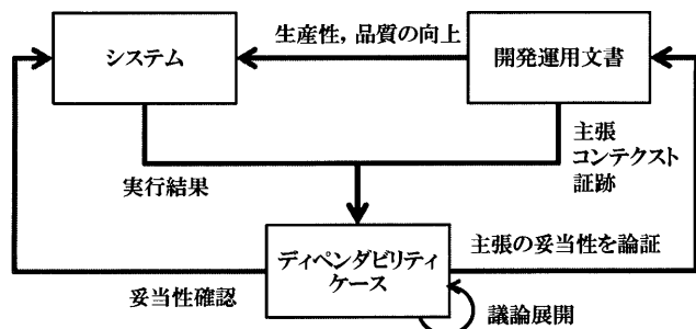
図3 システム、開発運用文書とディペンダビリティケースの関係
