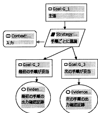
図4 プロセス定義に基づくディペンダビリティケース
