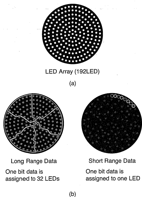
図 9 192 個の LED が同心円上に円形配置された場合の LED アレーの区分の一例 (a) LED アレー, (b) LED アレーの区分
