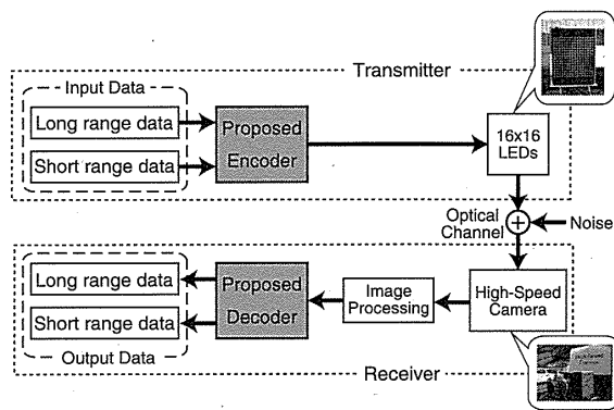
図 2 システムモデル Fig. 2 System model.
