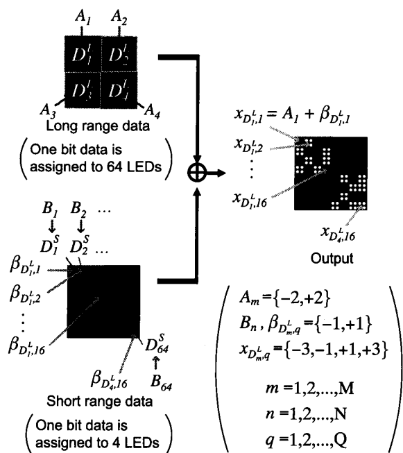
図6 符号化方式
