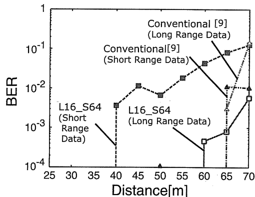
図 11 BER 特性 Fig. 11 BER performance.
