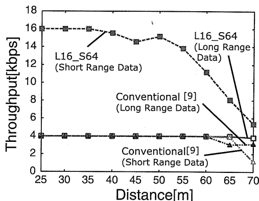
図 12 スループット特性 Fig. 12 Throughput performance.
