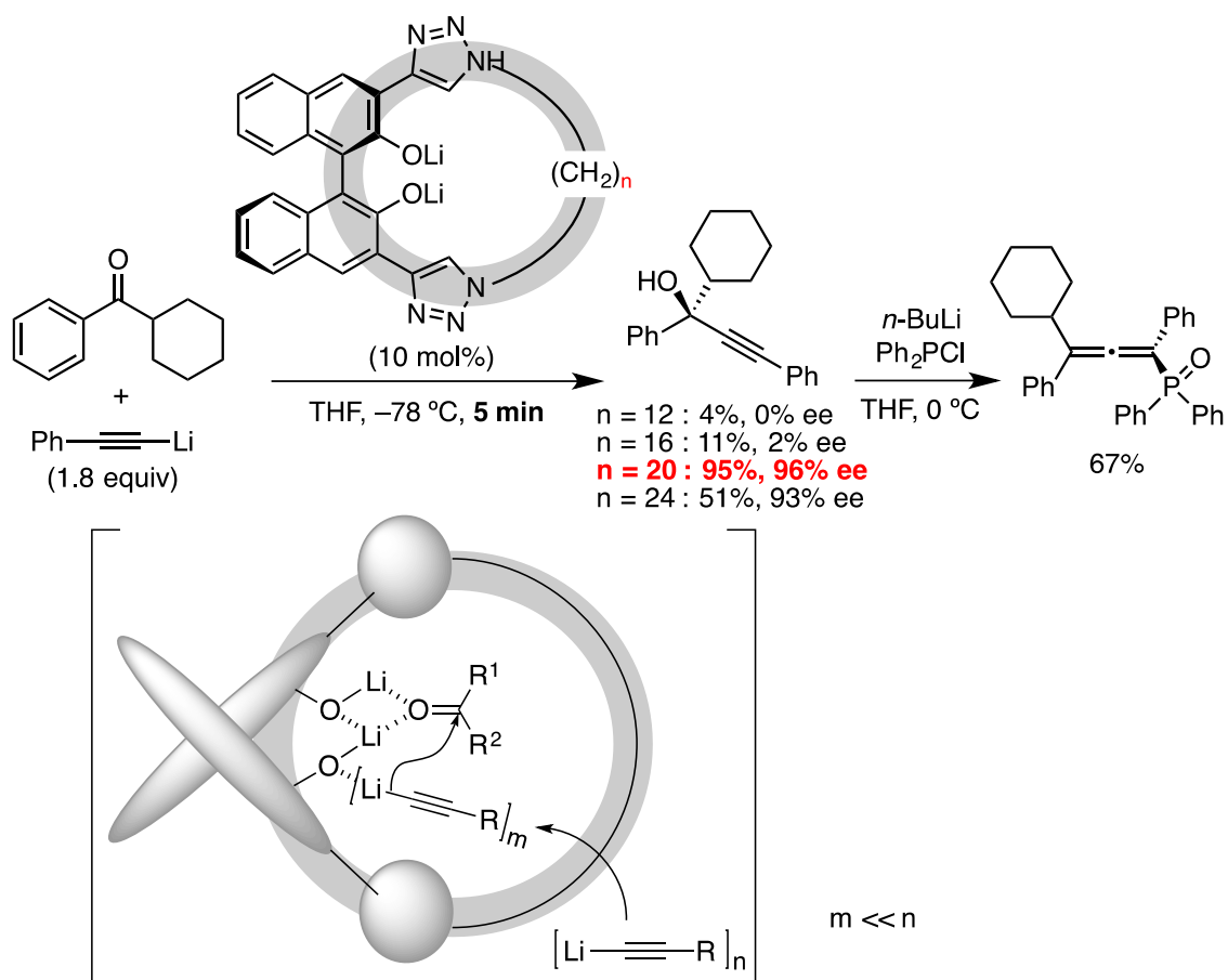
図 9: キラル大環状リチウム(I)ビナフトラート触媒を用いたケトンへのエナンチオ選択的アルキニル付加反応
