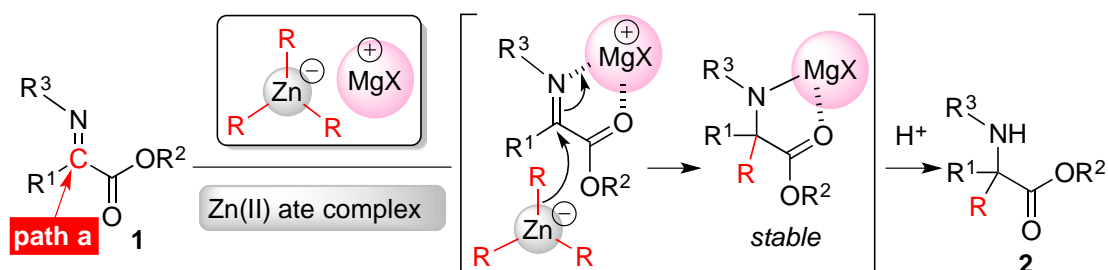
図 3: 想定される反応機構
