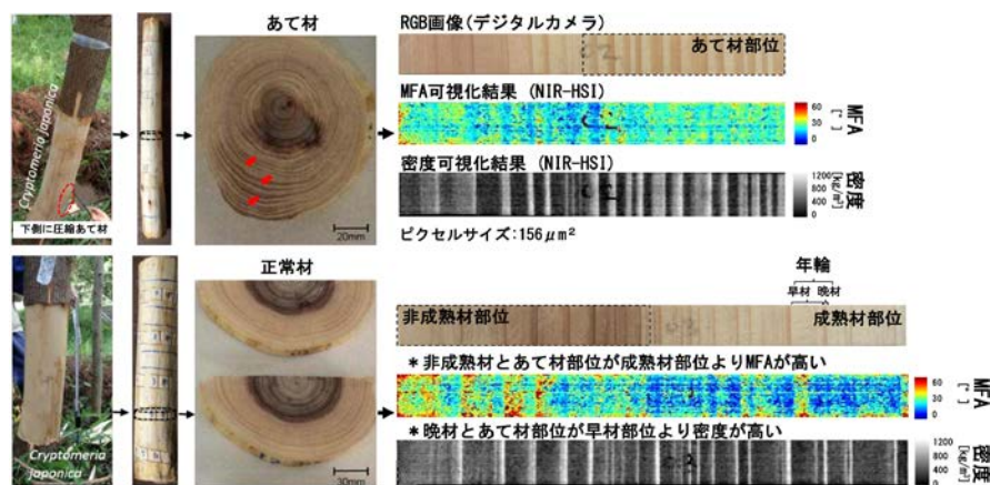
図 3. NIR-HSI法による木材密度およびマイクロフィブリル傾角(MFA)の可視化結果、晩材と“あて材”部位が早材部位より密度が高く、未成熟材と“あて材”部位が成熟材部位よりMFAが高いなど材の形成に伴う密度分布やMFA変動の違いが明瞭に確認可能
