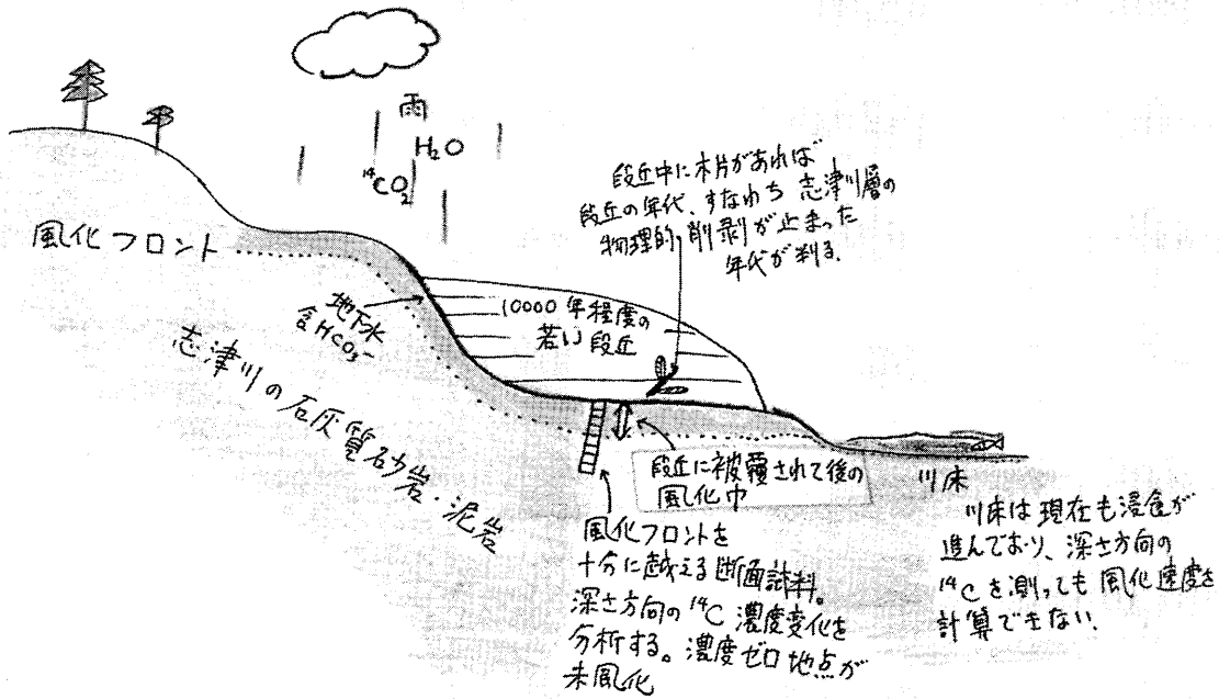
図 1 : 石灰質砂岩の風化断面を用いたコンクリート風化のナチュラルアナログの考え方。
