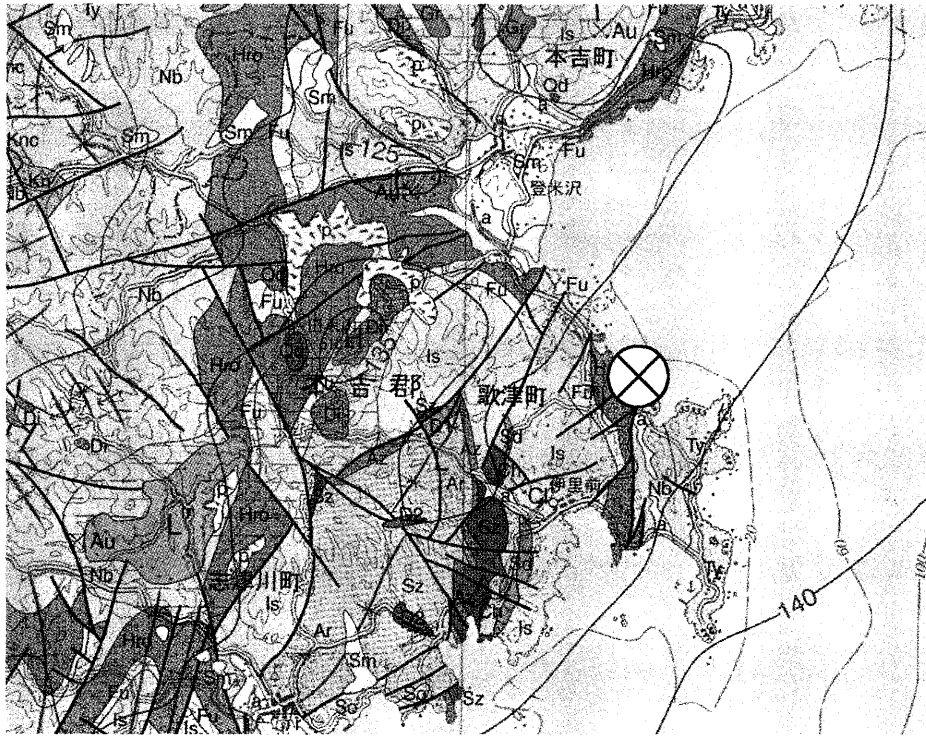
図 2 : 石灰質砂岩試料の採取地域の地質（竹内ほか、1/20 万 一関図幅）および採集地点。図中の紫色（Hro）部分が三疊紀稲井層群中の平磯層および大沢層の分布域を示す。
