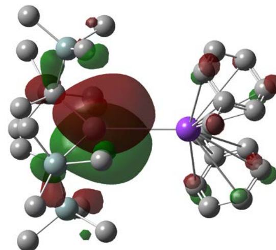
LUMO+8 (-0.1342 eV)
