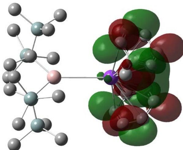
LUMO (-1.0667 eV)
