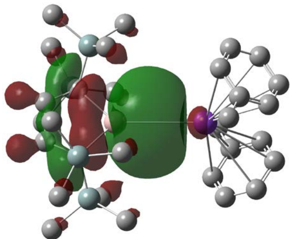
HOMO (-3.6303 eV)
