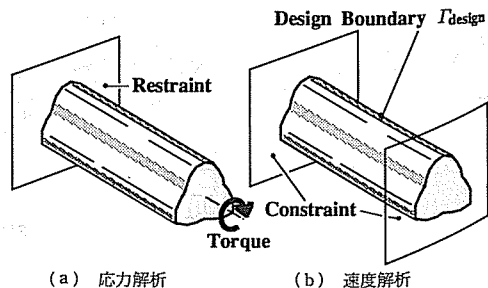
図9 トーションバの問題設定
