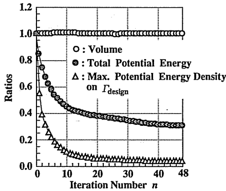
図 14 ブラケットの最適化履歴
