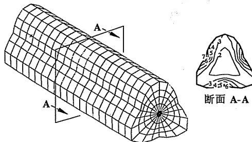
図10 トーションバの計算結果
