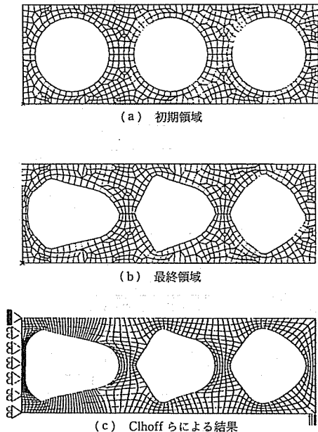
図7 有孔平板の計算結果
