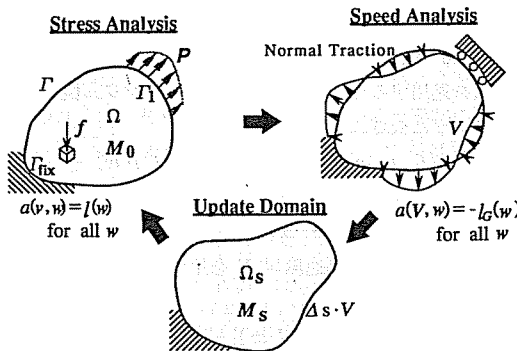
図2 方法の概念図
