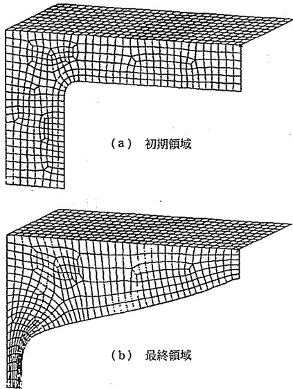
図 13 ブラケットの計算結果
