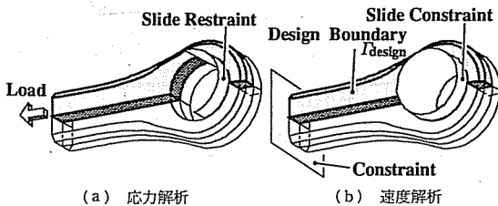
図 15 コンロッドの問題設定
