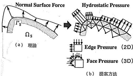
図4 汎用 FEM コードを利用した力法
