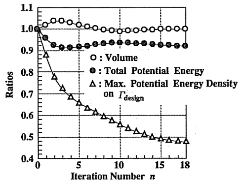
図11 トーションバの最適化履歴
