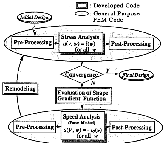
図5 領域最適化システム
