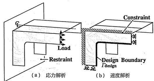
図12 ブラケットの問題設定
