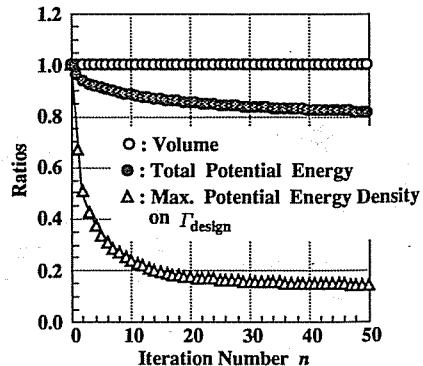
図 17 コンロッドの最適化履歴
