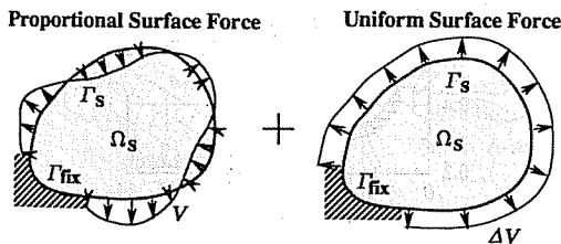
図3 体積制約を考慮した表面力
