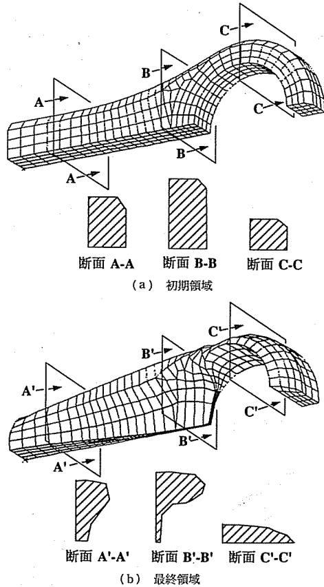
図 16 コンロッドの計算結果
