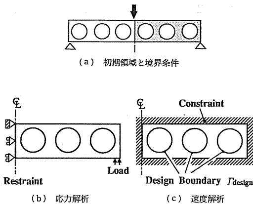
図6 有孔平板の問題設定
