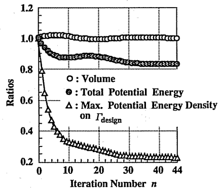
図8 有孔平板の最適化履歴
