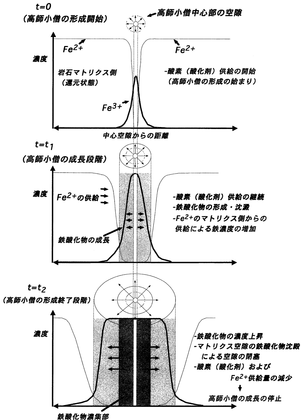
図3：高師小僧の無機化学反応プロセスのみによる形成過程モデル。ただし、無機化学反応は形成過程モデルでは、リング状の濃集形態や、外側ほど酸化鉄の濃集が高くなる高師小僧の形成過程を説明することはできない。
