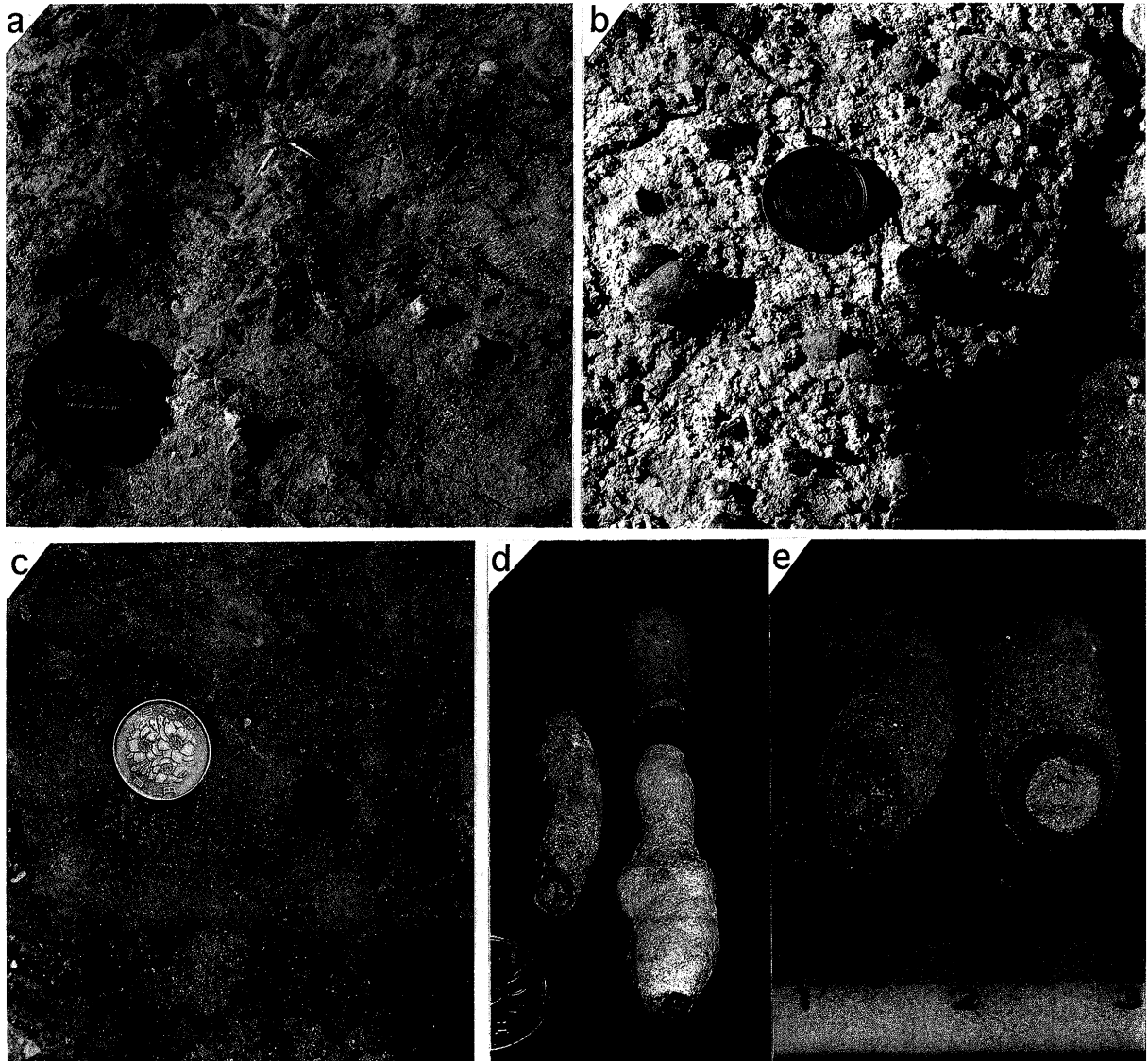
写真1：高師小僧の産状。a,b)斜面露頭での産状。地層中にはほぼ立った状態で産する。c)露頭での高師小僧断面。d)高師小僧の形態。棒状から凹凸のあるもの。また先端が丸くくびれたものなどが確認できる。e)高師小僧の断面構造。リング状の構造が確認できる。
