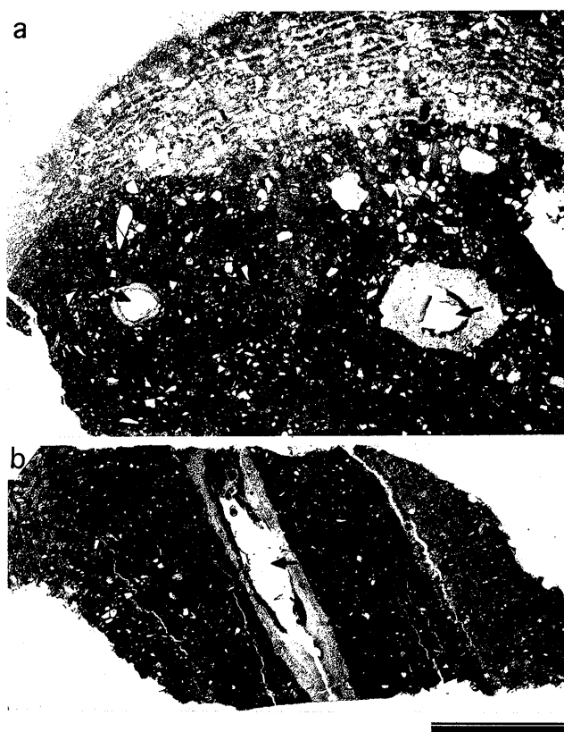
写真2：高師小僧の断面顕微鏡写真。a) 横断面構造。この高師小僧は、2つの空隙(矢印)の部分から1つのものに成長したものと思われる。外縁部分には、幅数十ミクロン程度の細かいリング構造が確認できる。b) 縦断面写真。中心部分の空隙(矢印)周辺には植物起源と思われる繊維組織が観察される(スケールは2mm)。
