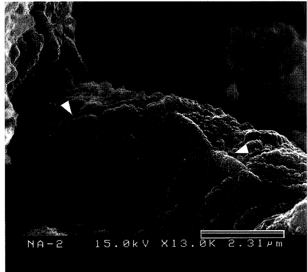
写真3：高師小僧の鉄酸化物中の微小空隙中で確認されたロッド状の微生物の痕跡(矢印)と思われる形態の電子顕微鏡写真。
