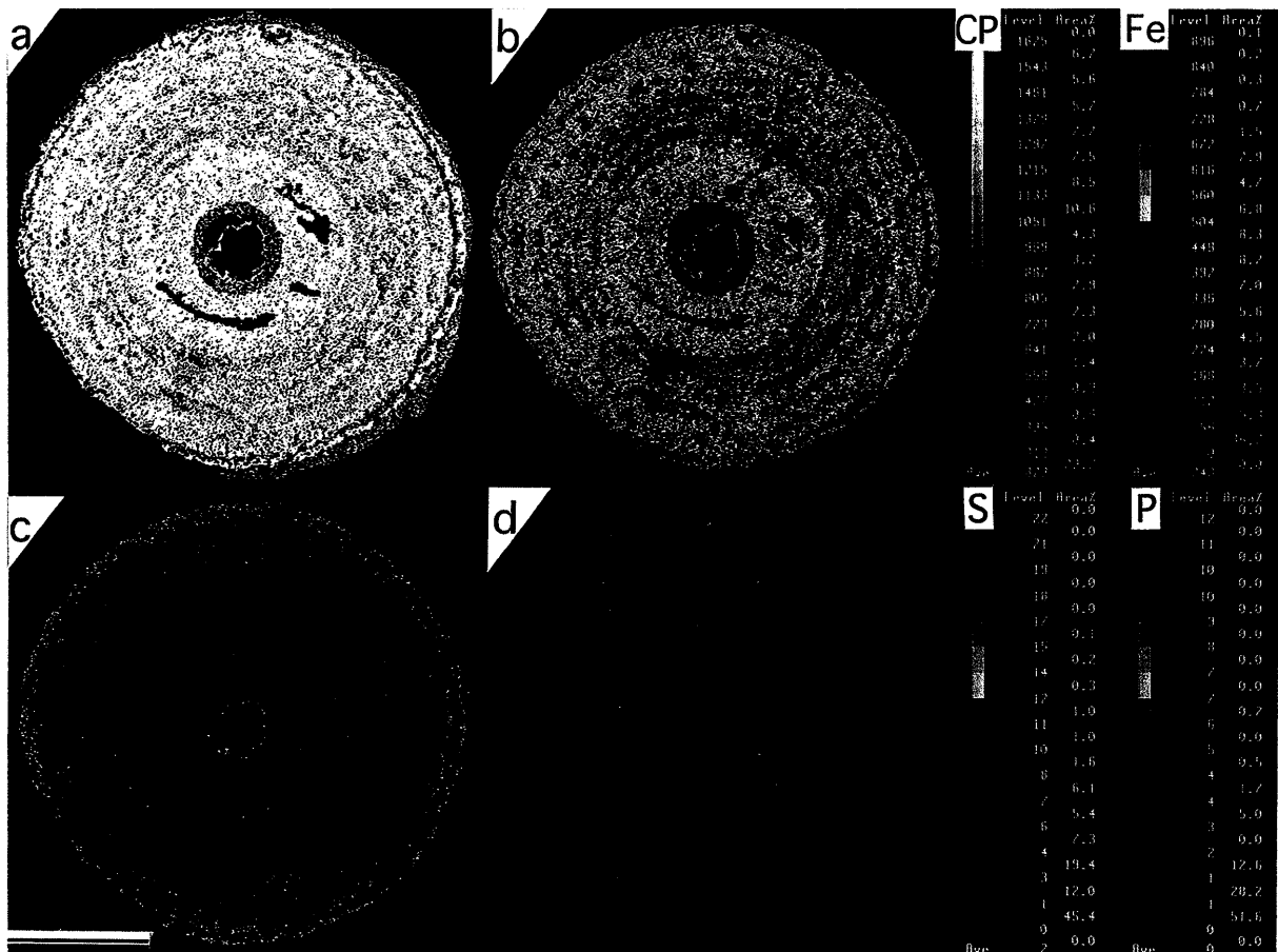
図1：高師小僧横断面の元素 (b：鉄 (Fe), c：硫黄 (S), d：リン (P)) およびCP (a：反射電子像) マップ。リング状の二次的な元素濃集が明瞭である。鉄ととくに硫黄については、外側に濃度の高い部分が確認できる (スケールは5 mm)。
