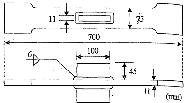
図-1 試験体の形状および寸法
