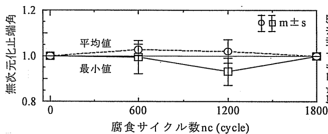
(c) 腐食前で腐食後を無次元化
