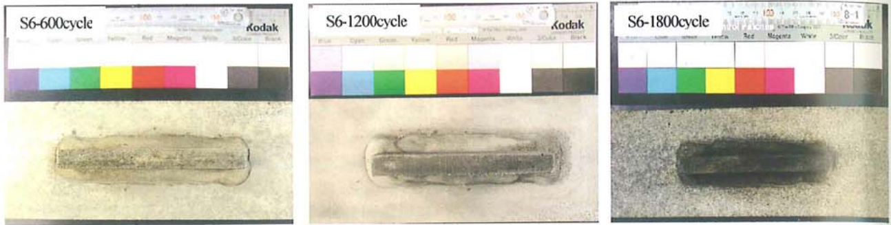
(b) さび除去後
