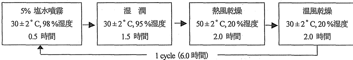
図-2 腐食促進試験の腐食促進サイクル
