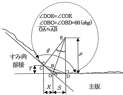
図4 止端角および止端半径の算出方法
