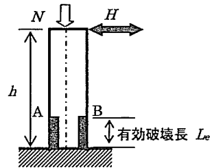
図-3 解析モデル概念図
