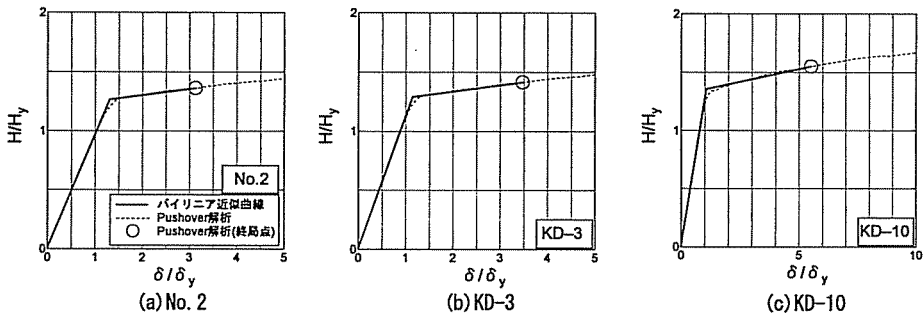
図-11 Pushover 解析結果，終局変位および推定復元力特性
