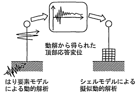
図-7 本解析手法概念図 (擬似動解)
