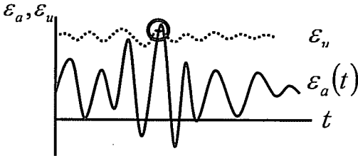
図-1 動的耐震照査法の概念図
