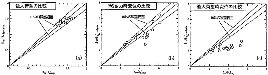
図-5 実験値と解析値の比較
