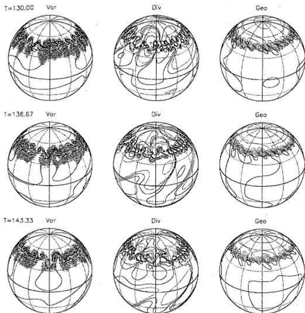
図3: 流れ場の時間発展の例。(左) 渦度 \zeta , (中) 発散 \delta , (右) ジオポテンシャルハイト \Phi である。渦度及び発散では負の領域に、ジオポテンシャルハイトでは平均水深以下の領域にハッチがかけてある。コンターは(左) 5 \times 10^{-5} 間隔, (中) \pm 10^{(-7, -6, -5, -4, -3)} , \pm 5 \times 10^{(-7, -6, -5, -4, -3)} , (右)31.6間隔(平均水深を基準として)で、正の値とゼロ値は実線、負の値は破線である。
