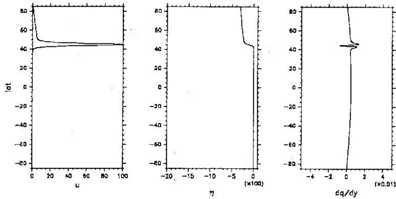
図 1: Ro = 10 , Fr = 0.7 における帯状な基本場の緯度構造の拡大図: (左) \bar{u}(\theta) , (中) \bar{q}(\theta) , (右) d\bar{q}(\theta)/d\theta .
