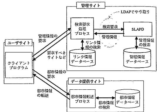
図 4 都市情報の検索処理の流れ
