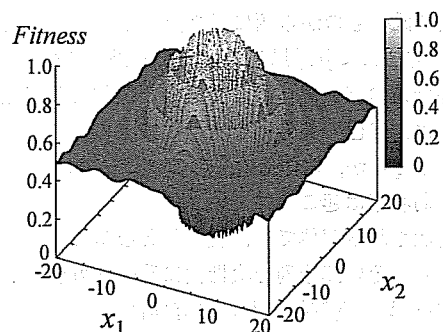
図2 SchafferのF1関数(2変数)の解空間
