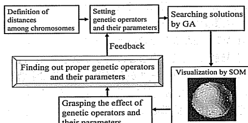
図1 可視化による遺伝的演算へのフィードバック Fig. 1 Feedback into genetic operators from visualization of search process.
