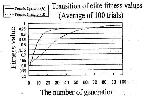
図 3 エリート評価値の推移
