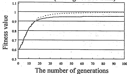
図 9 エリート評価値の推移
