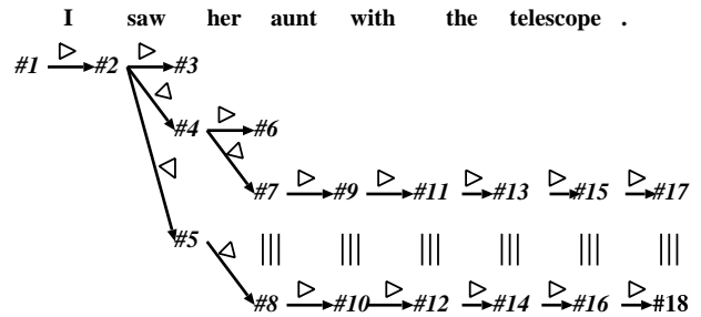
図 3: 項の間の包含関係 ▷* と同値関係 ≡
